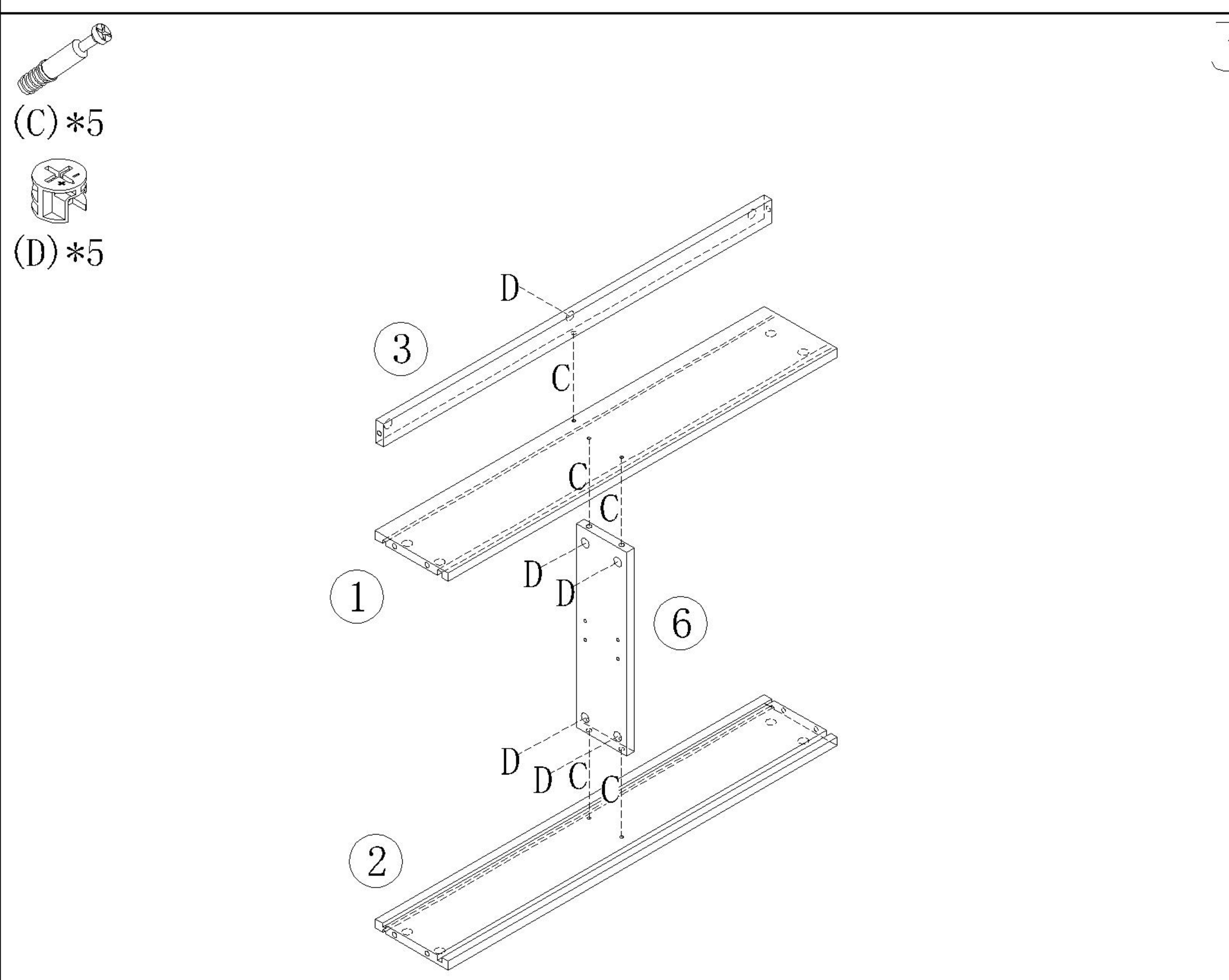
主轨 Main track
